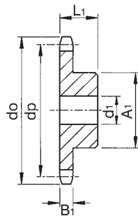
ANSI 25 (ISO Ref 04A)
