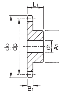
ANSI 41 (ISO Ref 085)
